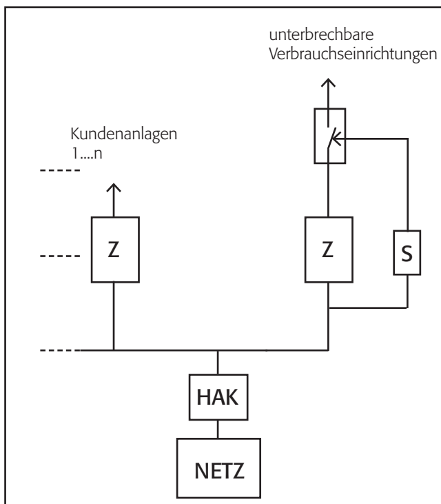
Bild1: Anschluss Nachtspeicheranlage
