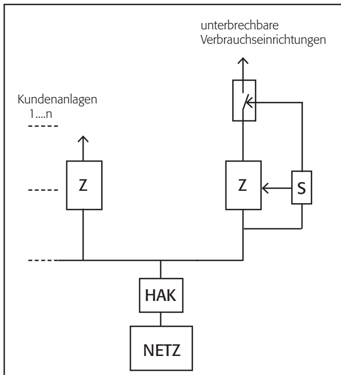
Bild1: Anschluss Wärmepumpenanlage
